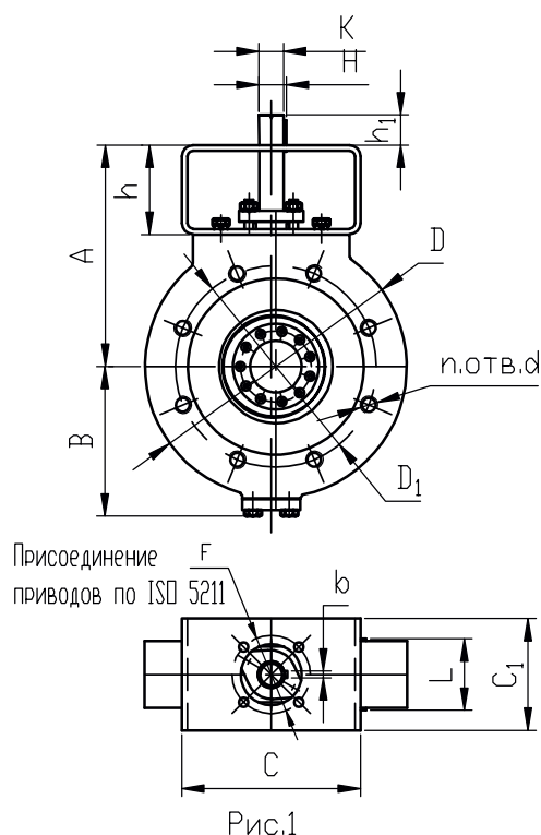
Рис. 1 – без привода Рис. 2 – с редуктором Рис. 3 – с электроприводом Рис. 4 – с пневмоприводом
